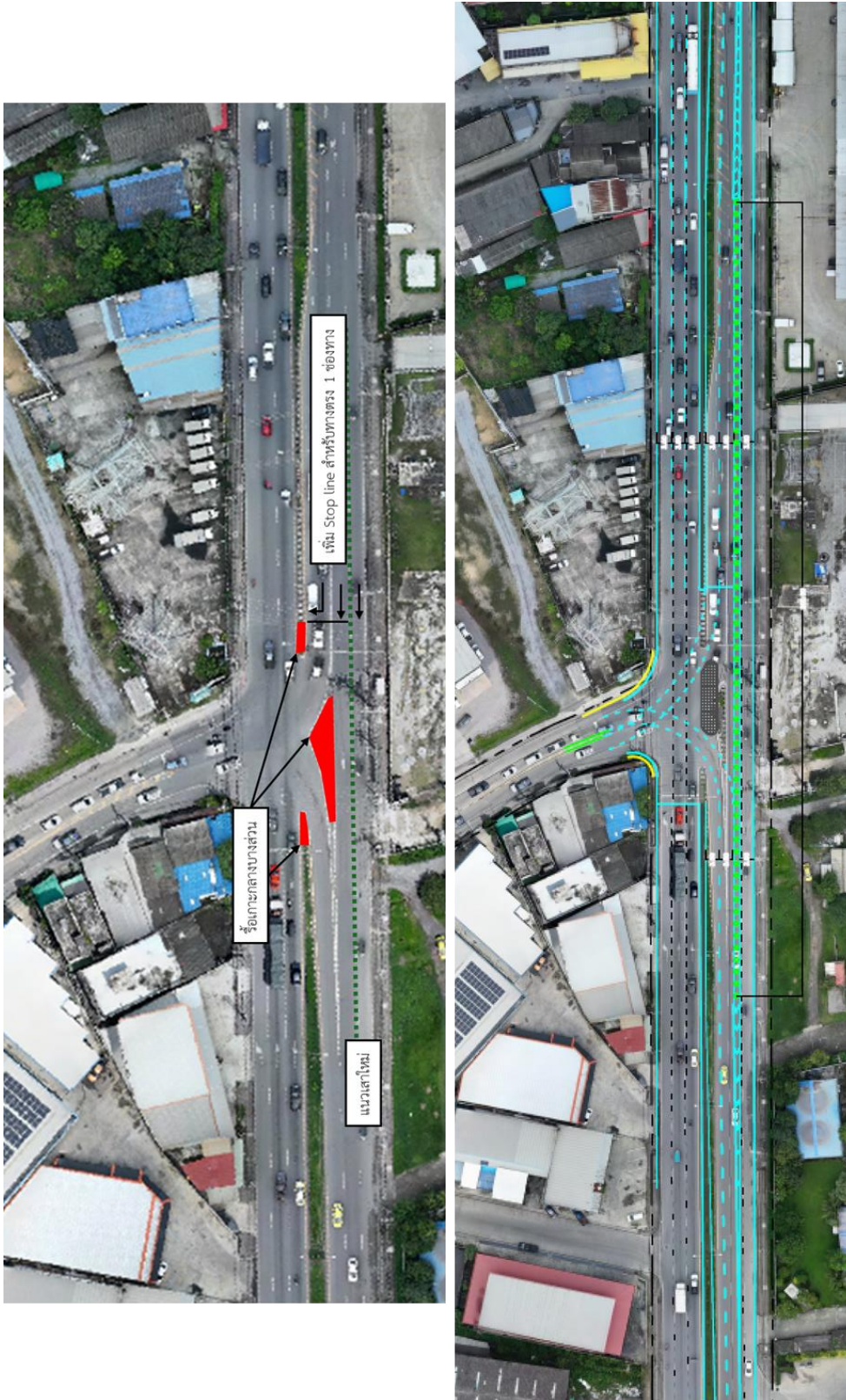
รูปที่ 10.1-5 แนวทางการแก้ไขปัญหาจราจรบริเวณแยกบางปลา
